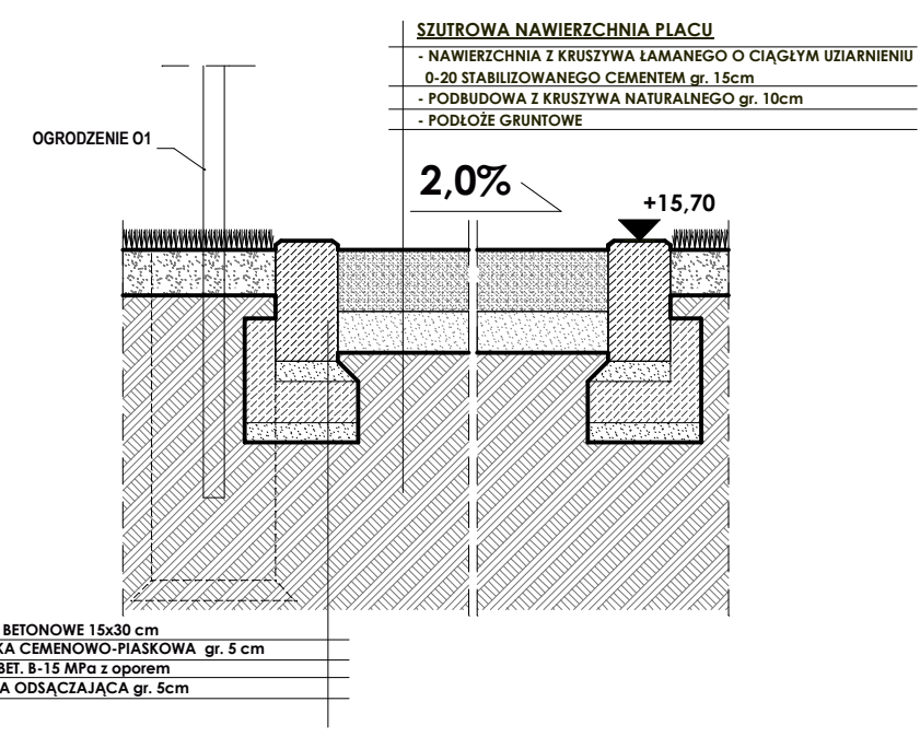
PRZEKRÓJ C-C PRZEZ PLAC O NAWIERZCHNI SZUTROWEJ
