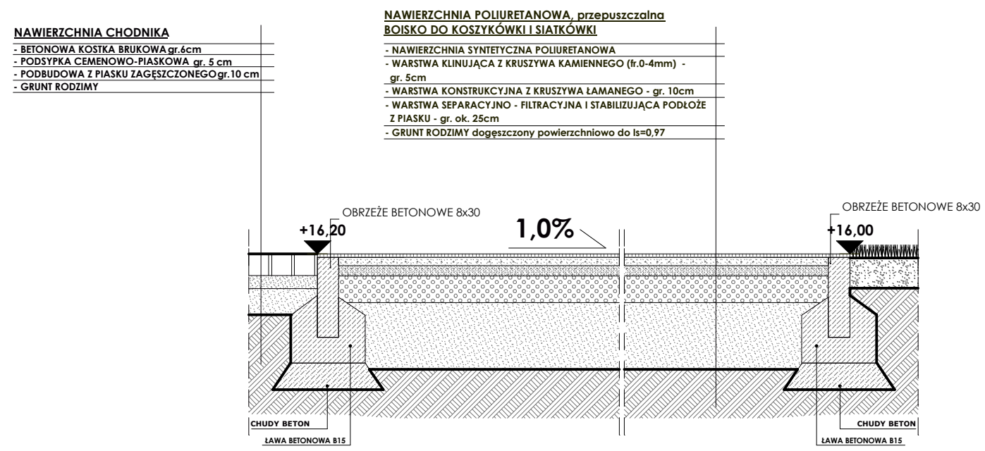
PRZEKRÓJ B-B PRZEZ BOISKO DO KOSZYKÓWKI I SIATKÓWKI
