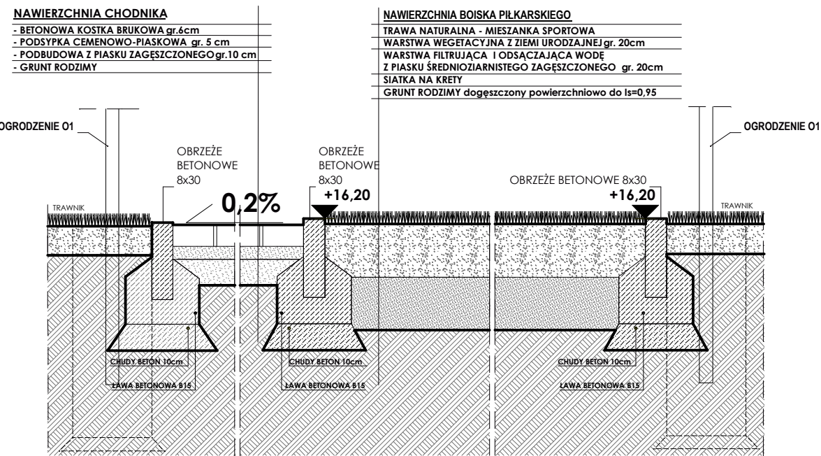
PRZEKRÓJ A-A PRZEZ BOISKO PIŁKARSKIE
